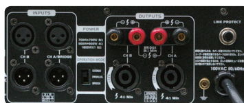
E-7500II リアパネル
